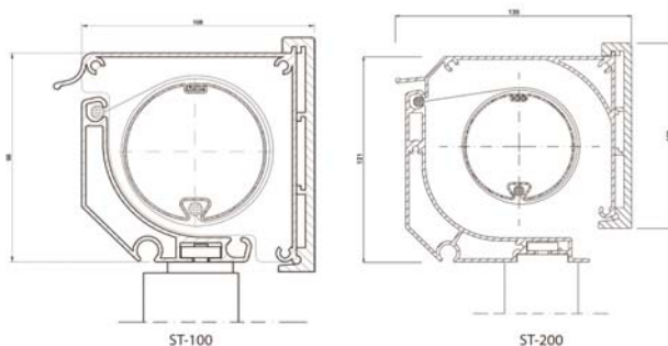
Tekening van de gesloten cassettevorm
